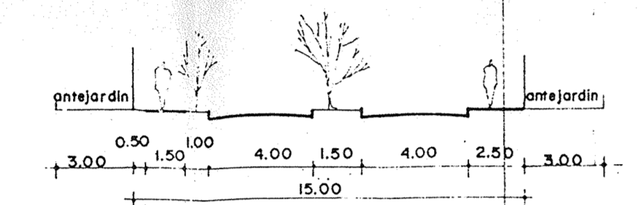
CORTE B-B' PASAJE DOCE ESC. 1:200
