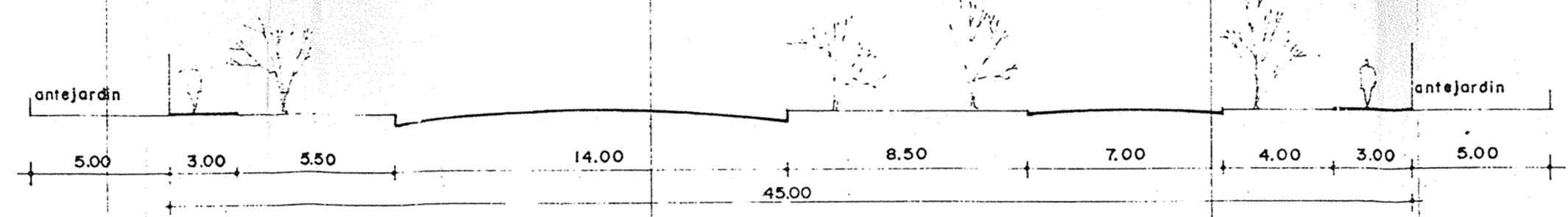
CORTE C-C' VICUÑA MACKENNA ORIENTE ESC. 1:200
