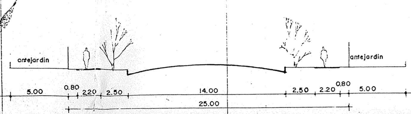
CORTE A-A' MIRADOR AZUL ESC. 1:200
